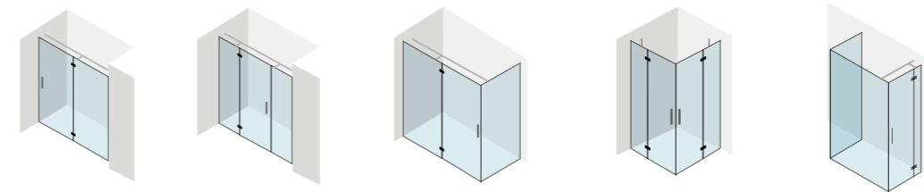
NICCHIA > Battente NICCHIA > Battente con porta centrale ANGOLO > Battente 1 porta + fisso laterale ANGOLO > Battente 2 porte PARETE > 3 lati Hinged door with in-line fixed panel Hinged door with 2 in-line fixed panels Hinged door with in-line fixed panel + fixed side panel 2 hinged doors with in-line fixed panels Hinged door with 2 fixed panels Porte battante avec paroi fixe alignée Porte battante avec 2 parois fixes alignées Porte battante avec paroi fixe alignée + côté fixe 2 portes battantes avec parois alignées Porte battante avec côté fixes
