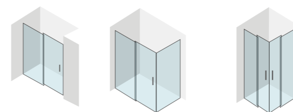
NICCHIA > Scorrevole ANGOLO > Scorrevole 1 porta + fisso laterale ANGOLO > Scorrevole 2 porte 1 sliding door 1 sliding door + fixed panel 2 sliding doors Porte coulissante Porte coulissante + côté fixe 2 portes coulissantes
