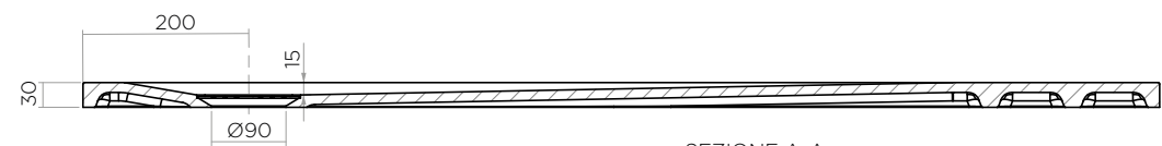
SEZIONE A-A
