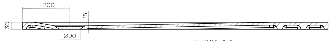
SEZIONE A-A
