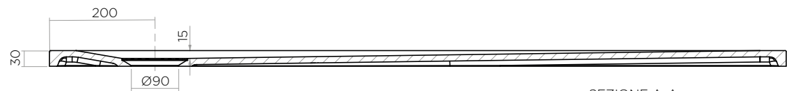
SEZIONE A-A
