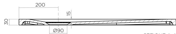
SEZIONE A-A
