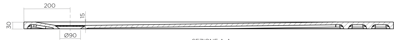
SEZIONE A-A
